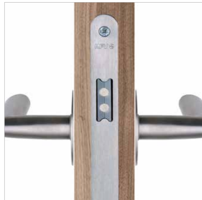
Das Magnetfallenschloss überzeugt durch eine leise Akustik und seine elegante Optik.
